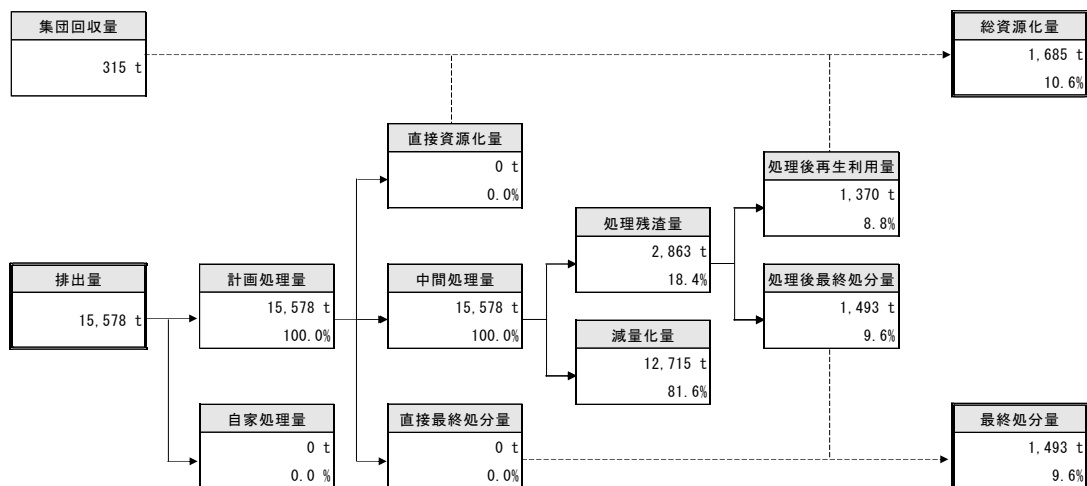
図 2-1 一般廃棄物の処理状況フロー
